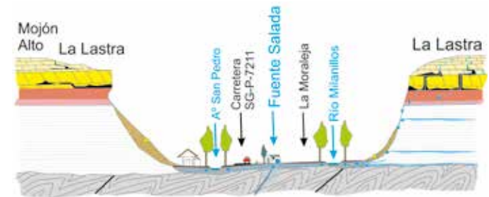
Corte hidrogeológico idealizado transversal al valle del río Milanillos, con la disposición de los diferentes acuíferos y acuitardos que pueden estar relacionados con la Fuente Salada.
