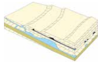
Proceso de formación de una red de cavidades subterráneas por acción kárstica.
